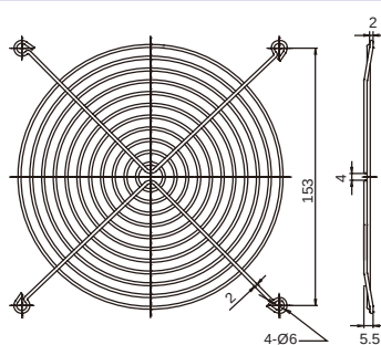
FG-18A For 176mm Fan
