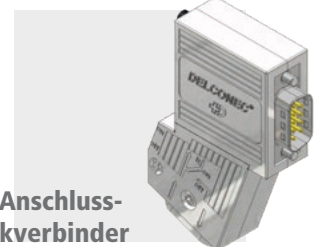
D-Sub Gehäuse
